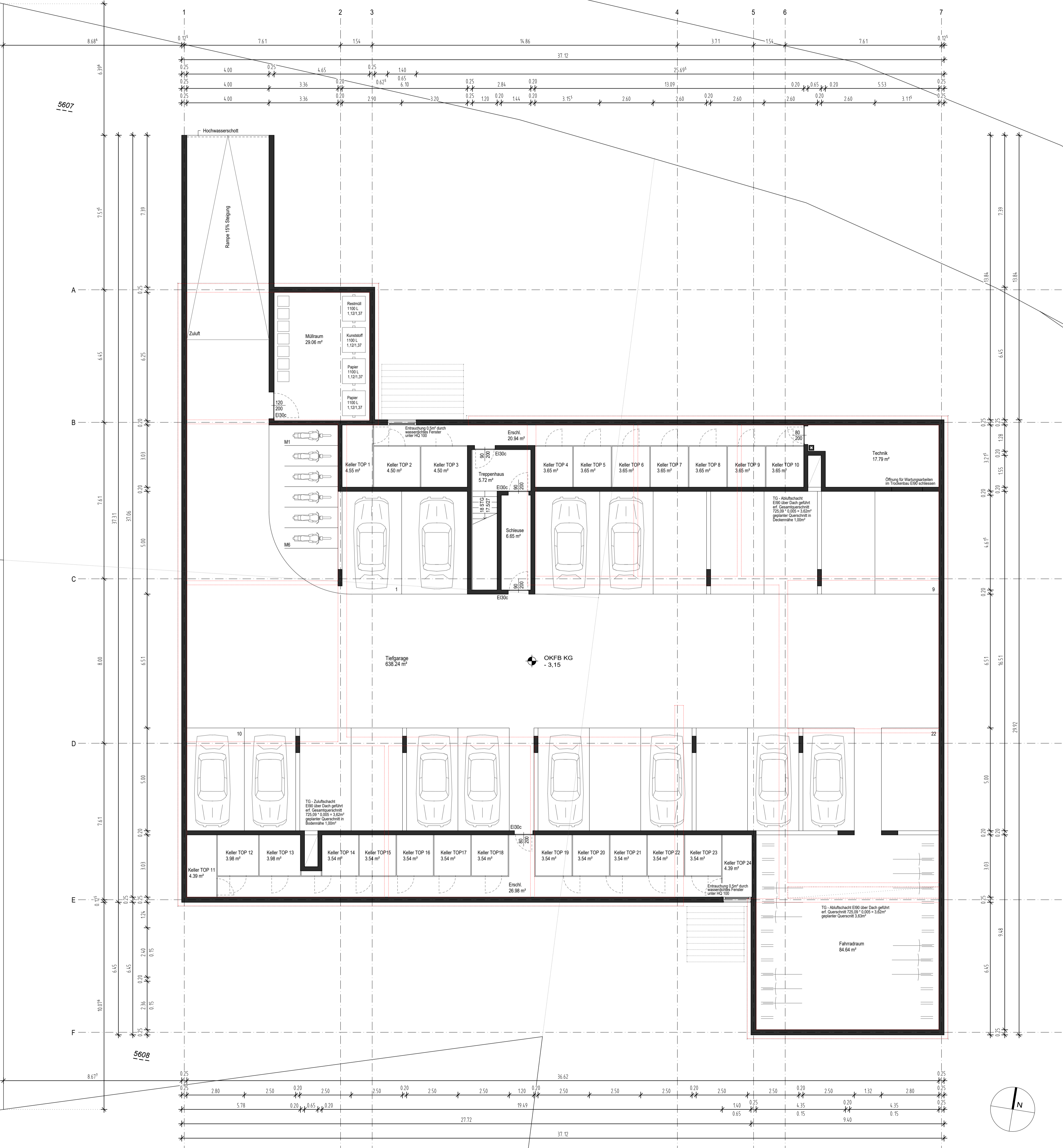
KELLERGESCHOSS 1/1000
